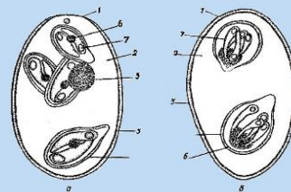
ооцист сызбасы
